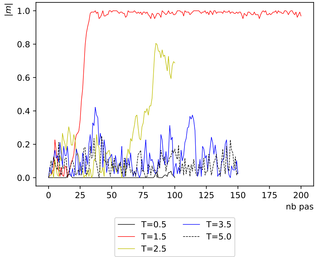
Evolution selon critère Estimation par intervalle,Condition Initiale alterné 4lignes-4lignes, Réseau taille L=16
